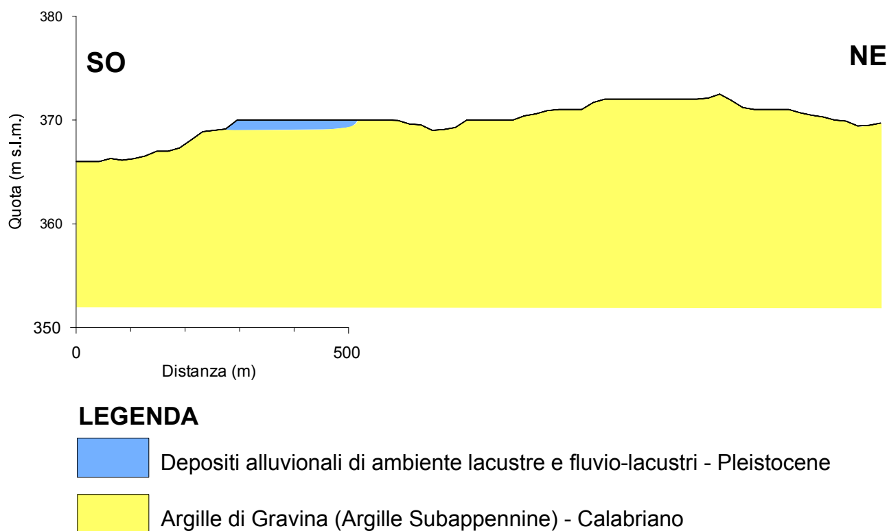
Figura 2.1.2 Stralcio di sezione geologica schematica dell'area TA_MT-17, traccia di sezione in Tavola 1.
