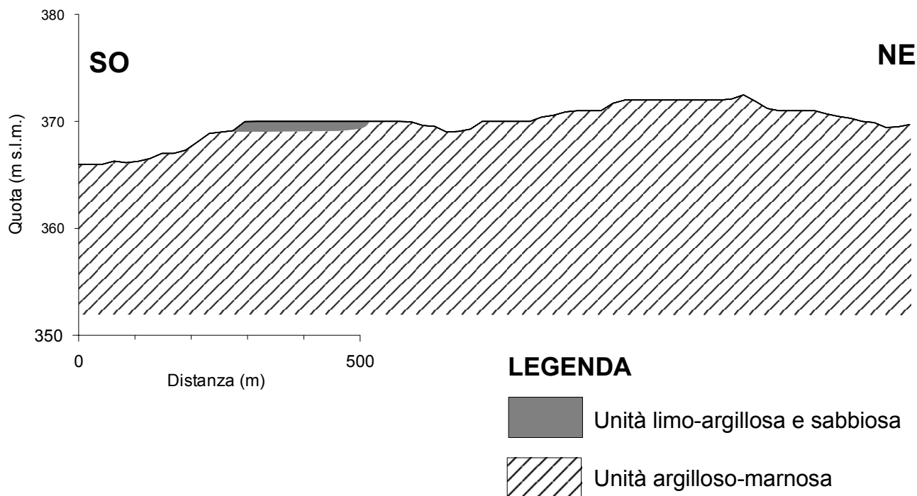
Figura 2.6.1 Schema geologico-tecnico dell'area TA_MT-17.
