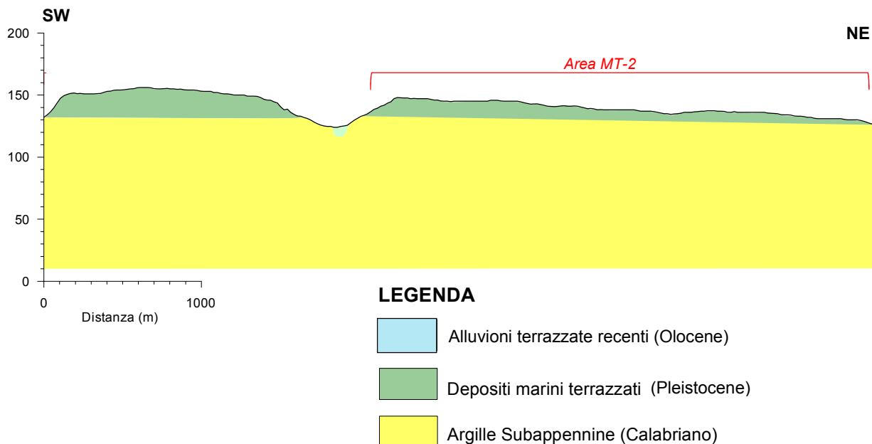
Figura 2.1.3 Sezione litostratigrafica schematica dell'area MT-2.
