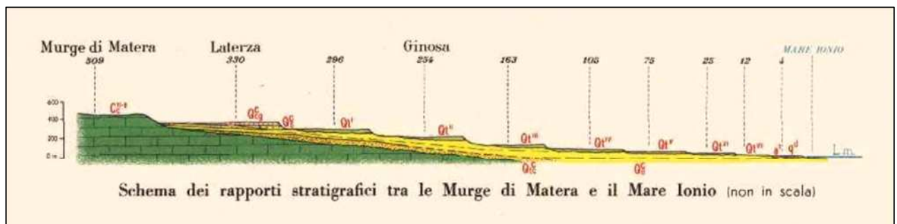
Figura 2.1.2 Schema dei rapporti stratigrafici del Foglio 201 "Matera" della Carta Geologica d'Italia (scala 1:100.000). Tale schema, seppur tratto da un foglio geologico differente da quello relativo all'area MT-2, permette di schematizzare i rapporti tra i depositi terrazzati del ciclo regressivo e le sottostanti unità plio-pleistoceniche.
