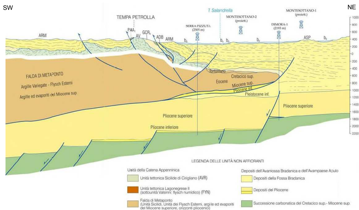
Figura 2.1.1 Stralcio di sezione stratigrafica tratta dal Foglio 507 "Pisticci" (1:50.000), modificata. L'area MT-2 può essere proiettata in prossimità del pozzo "Serra Pizzuta".
