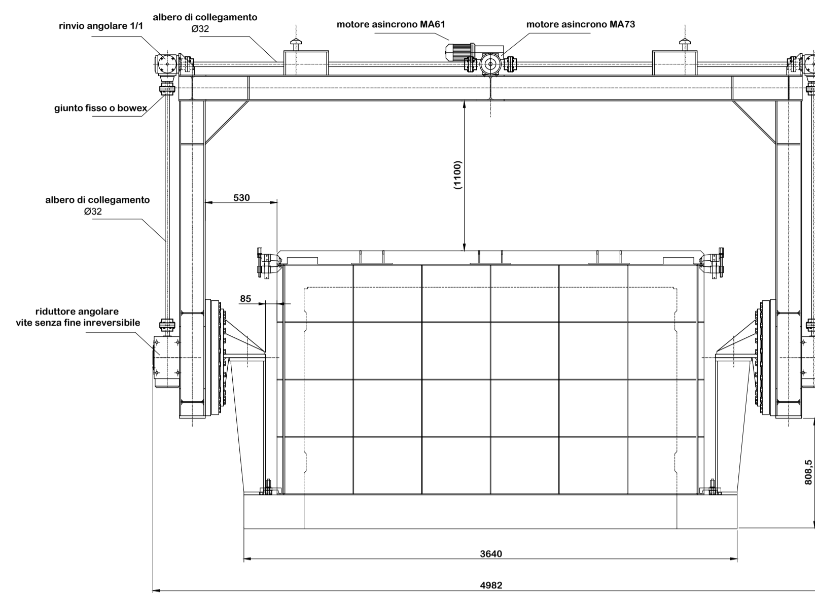
VISTA LONGITUDINALE
