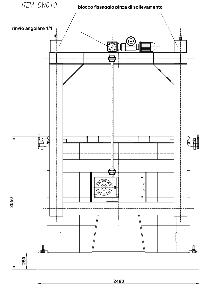
VISTA TRASVERSALE
