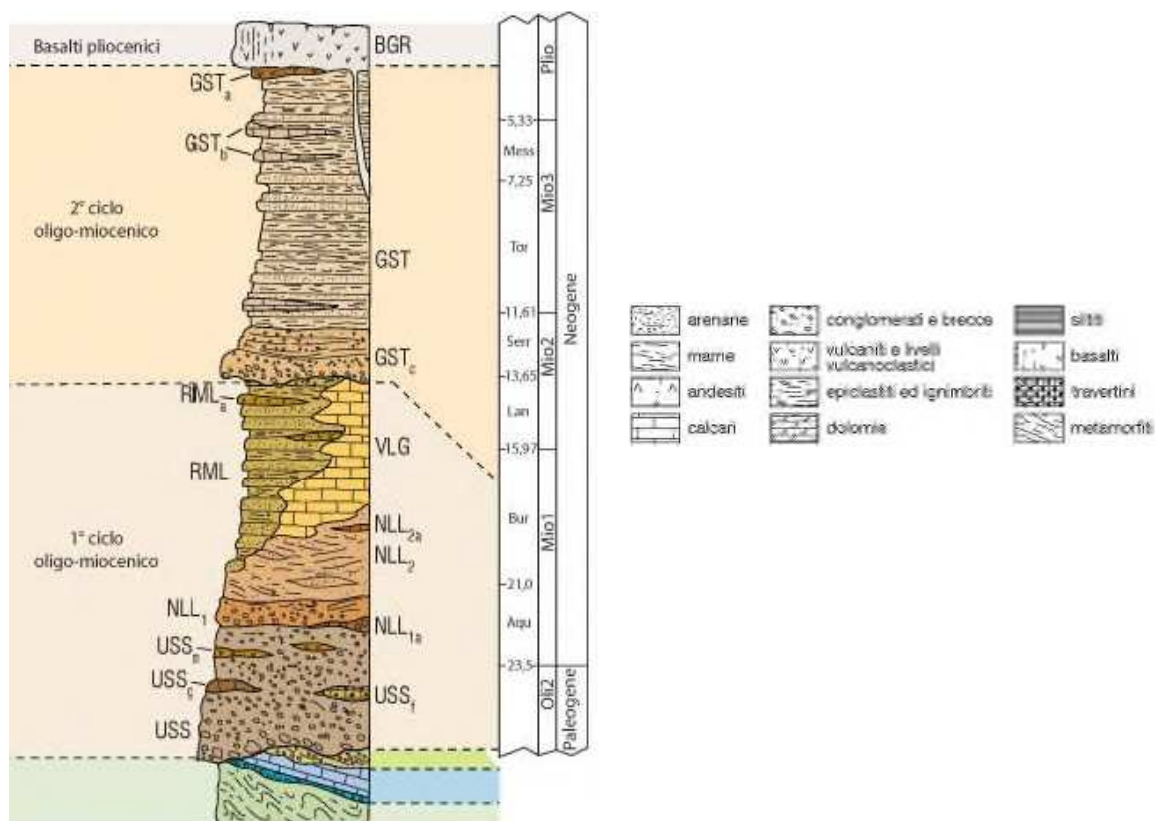
Figura 2.1.2 Colonna litostratigrafica delle successioni permiane, mesozoiche e terziarie, da Foglio 540 "Mandas".
