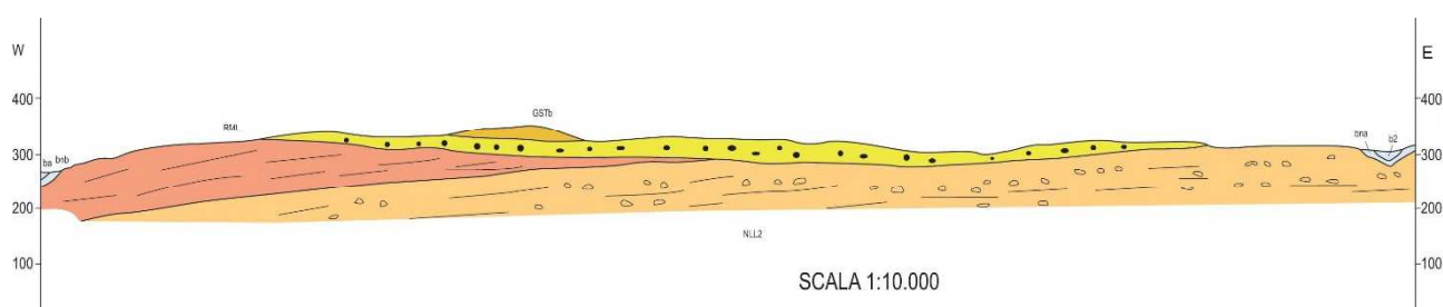
Figura 2.1.3 Sezione litostratigrafica con direzione Ovest-Est dell'area SU-64; la traccia di sezione è riportata in Tavola 1.
