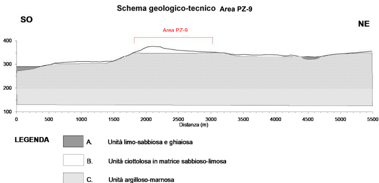
Figura 2.6.1 Schema geologico-tecnico dell'area PZ-9.
