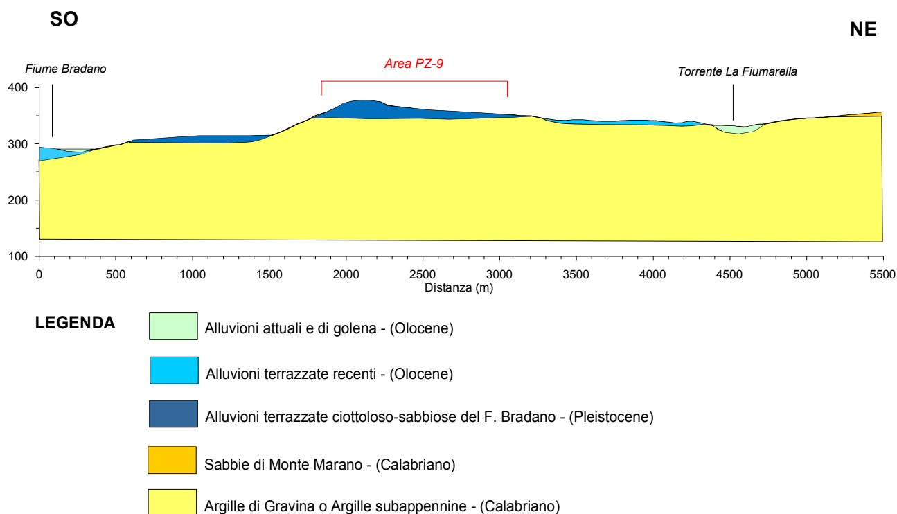
Figura 2.1.2 Sezione geologica schematica dell'area PZ-9.
