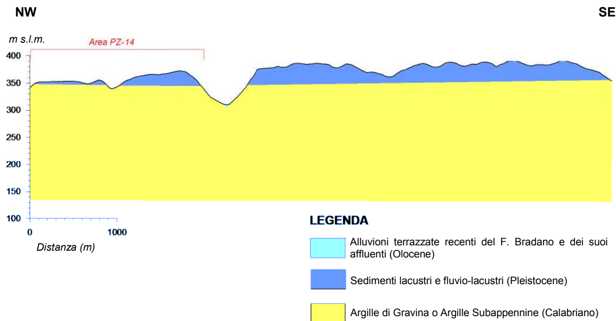
Figura 2.1.2 Sezione geolitologica dell'area PZ-14.
