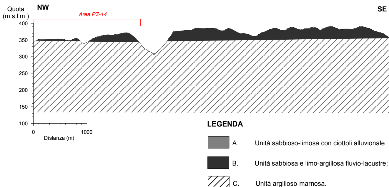
Figura 2.6.1 Schema geologico-tecnico dell'area PZ-14.
