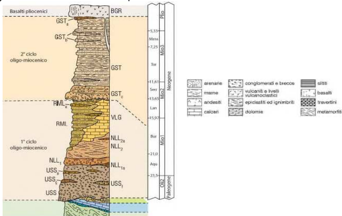
Figura 2.1.2 Colonna litostratigrafica delle successioni paleozoiche, mesozoiche e terziarie, da Foglio 540 "Mandas".
