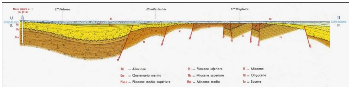
Figura 2.1.1 Sezione II del Foglio Geologico 70 "Alessandria" rappresentante l'alto strutturale pre-pliocenico sepolto dalle coperture quaternarie.
